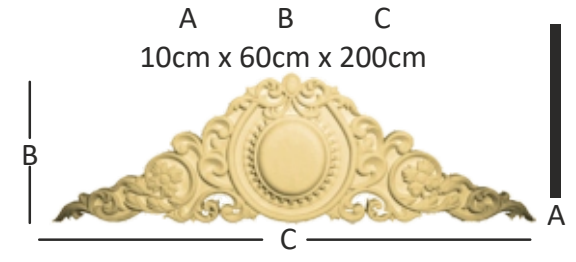
ADT - 04 DESENLİ TAÇ
