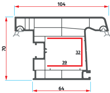
ER 7022 Dışa Açılır Kapı Kanat Profili Transom Door Sash Profile
