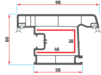
ER 6006 Dışa Açılır Kapı Kanat Profili Transom Door Sash Profile
