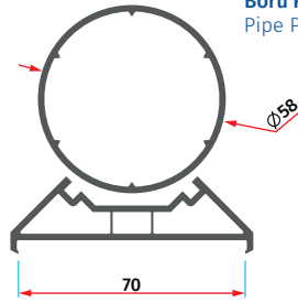
ER 7007 70'lik Dönüş Adaptörü 70 Pipe Return Profile
