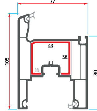
S - 1040 Sürme Kanat Profili Sliding Sash Profile
