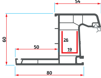
ER 6003 Pervazlı Kasa Profili Frame with Cornice Profile
