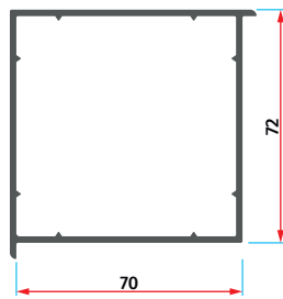
ER 7006 Kutu Profili 70x70 Box Profile 70x70
