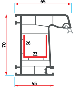
ER 7010 Kasa Profili Frame Profile
