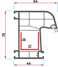
ER 7018 Oval Kasa Profili Ovoid Frame Profile
