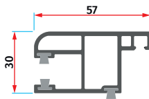
S - 1023 Sürme Sineklik Kanat Sliding Screened Sash
