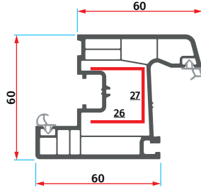
ER 6004 Pencere Kanat Profili Window Sash Profile
