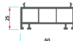
ER 6032 60'lik Kasa Yükseltme 60 Frame Lift
