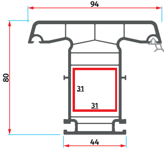
S - 1041 Sürme Orta Kayıt Profili Sliding Mullion Profile
