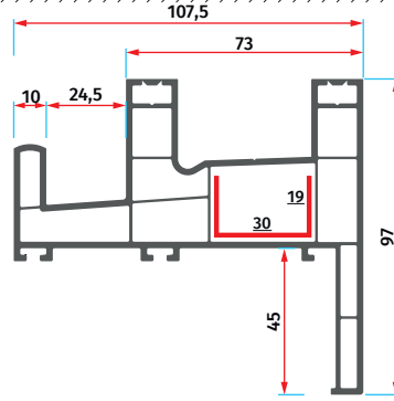
S - 1020 Sürme Sineklikli Çiftli Pervazlı Kasa Sliding Screen Double Frame with Cornice
