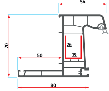
ER 7012 Pervazlı Kasa Profili Frame with Cornice Profile
