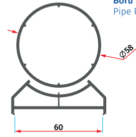
ER 6012 60'lik Dönüş Adaptörü 60 Pipe Return Profile
