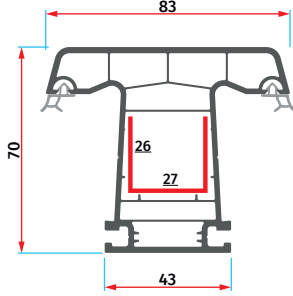
ER 7011 Orta Kayıt Profili Mullion Profile
