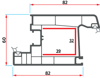
ER 6021 Kapı Kanat Profili Door Sash Profile
