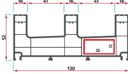
S - 1030 Sürme Üçlü Kasa Sliding Triple Frame
