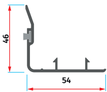
S - 1029 Sürme Kilit Adaptrörü Wide Sash Closing
