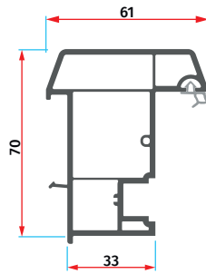
ER 7021 70'lık Hareketli Orta Kayıt Profili 70 Movable Mullion Profile
