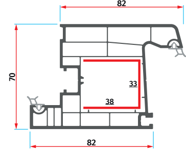
ER 7014 Kapı Kanat Profili Door Sash Profile
