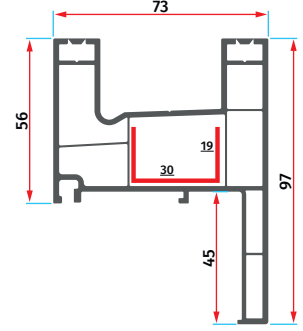
S - 1026 Sürme Çiftli Pervazlı Kasa Sliding Double Frame with Cornice
