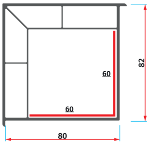
ER 8012 Kutu Profili 80x80 Box Profile 80x80
