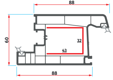
ER 6005 Kapı Kanat Profili Door Sash Profile
