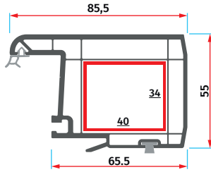
S - 1025 Dikey Sürme Orta Kayıt Vertical Sliding Mullion
