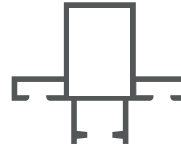
AKS 021 / 022 Sürme Alm. Birleştirme Sliding Sash Connection
