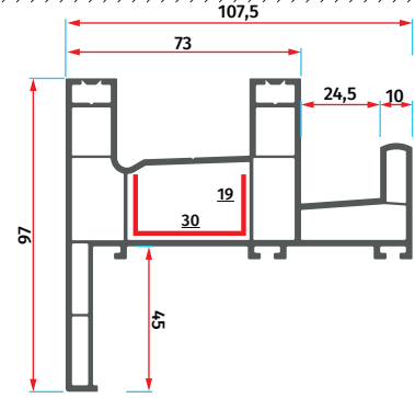
S - 1038 Ters Sürme Sineklikli Çiftli Pervazlı Kasa Reverse Sliding Screen Double Frame with Cornice
