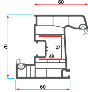
ER 7013 Pencere Kanat Profili Window Sash Profile
