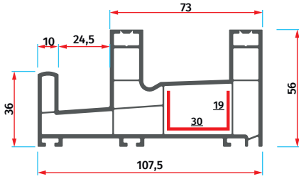
S - 1036 Sürme Sineklikli Çiftli Kasa Sliding Double Frame with Screen
