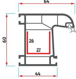
ER 6022 Oval Kasa Profili Ovoid Frame Profile
