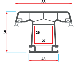
ER 6002 Orta Kayıt Profili Mullion Profile
