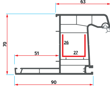
ER 7026 Geniş Pervazlı Kasa Profili Wide Frame with Cornice Profile
