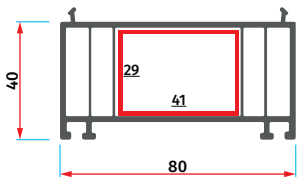
ER 8013 80'lik Kasa Yükseltme 80 Frame Lift
