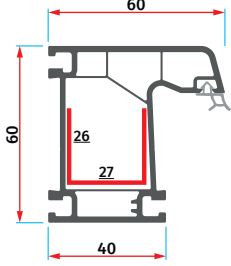
ER 6018 Kasa Profili Frame Profile
