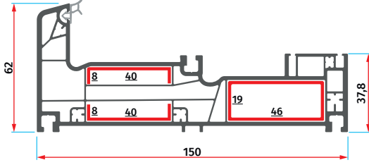
S - 1039 Sürme Kasa Profili Sliding Frame Profile
