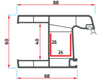
ER 6034 40'lık U Kasa Profili 40'lık U Frame Profile
