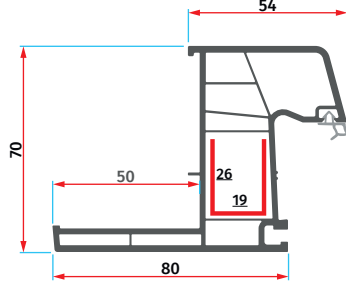
ER 7005 Pervazlı Kasa Profili Frame with Cornice Profile
