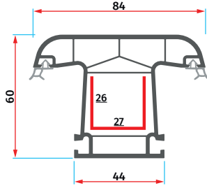
ER 6023 Oval Orta Kayıt Profili Ovoid Mullion Profile
