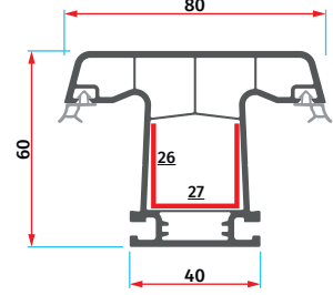
ER 6019 Orta Kayıt Profili Mullion Profile
