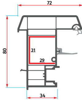
ER 8006 80'lık Hareketli Orta Kayıt Profili 80 Movable Mullion Profile
