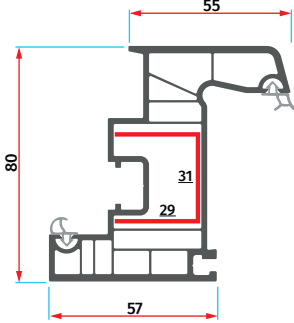
ER 8003 Pencere Kanat Profili Window Sash Profile
