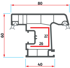
ER 6031 Dışa Açılır Pencere Kanat Profili Transom Window Sash Profile
