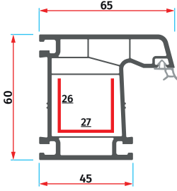
ER 6001 Kasa Profili Frame Profile
