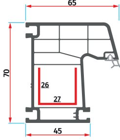
ER 7001 Kasa Profili Frame Profile
