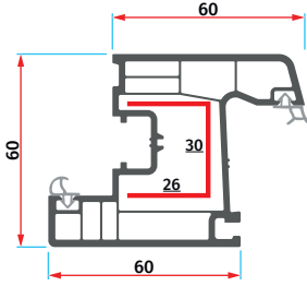
ER 6004 Pencere Kanat Profili Window Sash Profile
