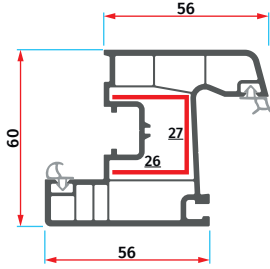
ER 6020 Pencere Kanat Profili Window Sash Profile
