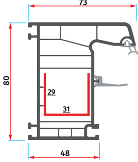
ER 8001 Kasa Profili Frame Profile
