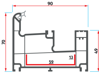
S - 1027 Sürme Tekli Kasa Sliding Single Frame
