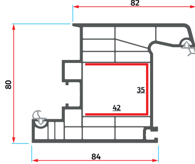
ER 8004 Kapı Kanat Profili Door Sash Profile
