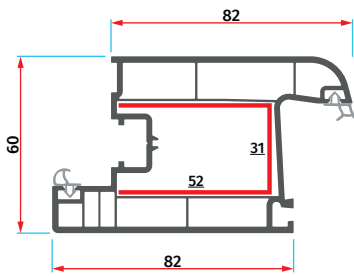
ER 6025 Oval Kapı Kanat Profili Ovoid Door Sash Profile
