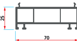
ER 7024 70'lik Kasa Yükseltme 70 Frame Lift
