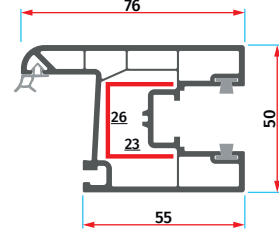
S - 1019 Sürme Kanat Sliding Window Sash
