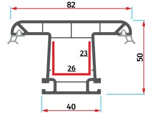
S - 1034 Sürme Orta Kayıt Sliding Mullion
