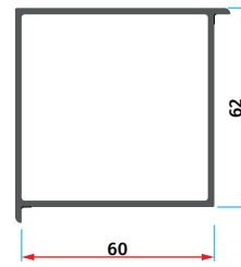
ER 6014 Kutu Profili 60x60 Box Profile 60x60
