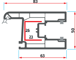
S - 1028 Geniş Sürme Kanat Wide Sliding Window Sash
